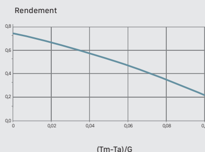
COURBE DE RENDEMENT INSTANTANÉE
