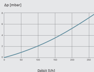
COURBE DE PERTE DE CHARGE
